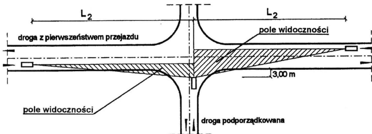
Rys. 3. Pole widoczności przy ruszaniu z miejsca zatrzymania
