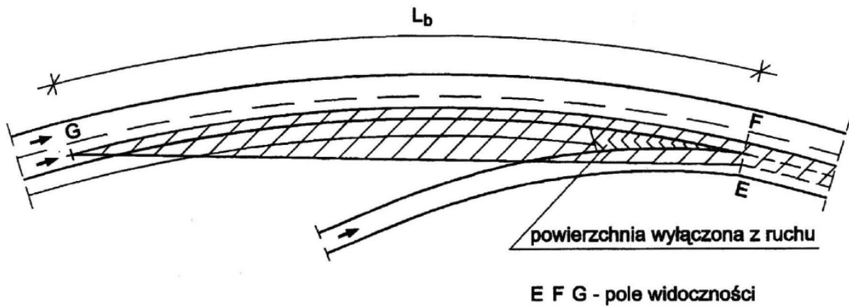
Rys. 2. Pole widoczności na pasie włączania
